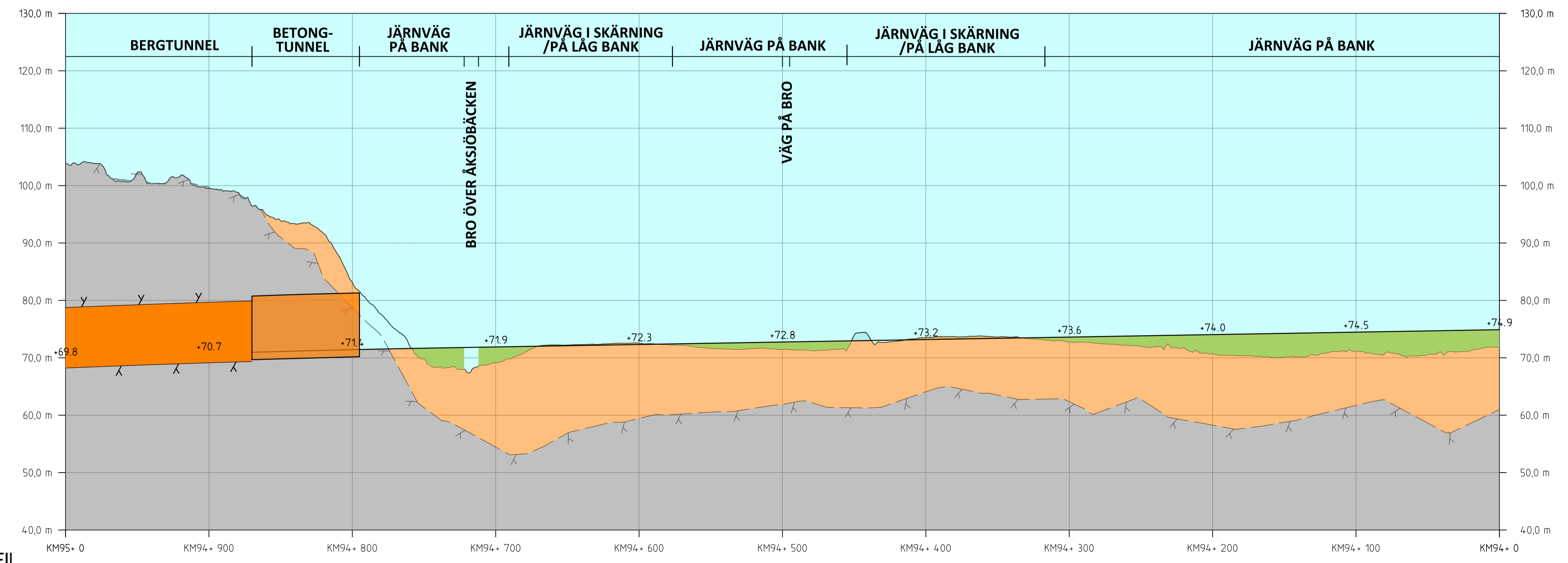
PROFIL SPÅRPROFIL LÅNGS NEDSPÅRET (ÖSTLIGA SPÅRET)
